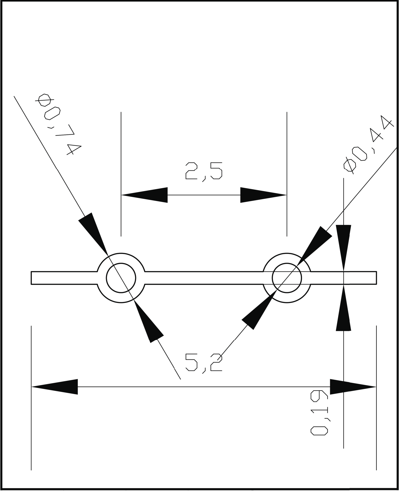
TWIST-BAND 2 X 0.44
