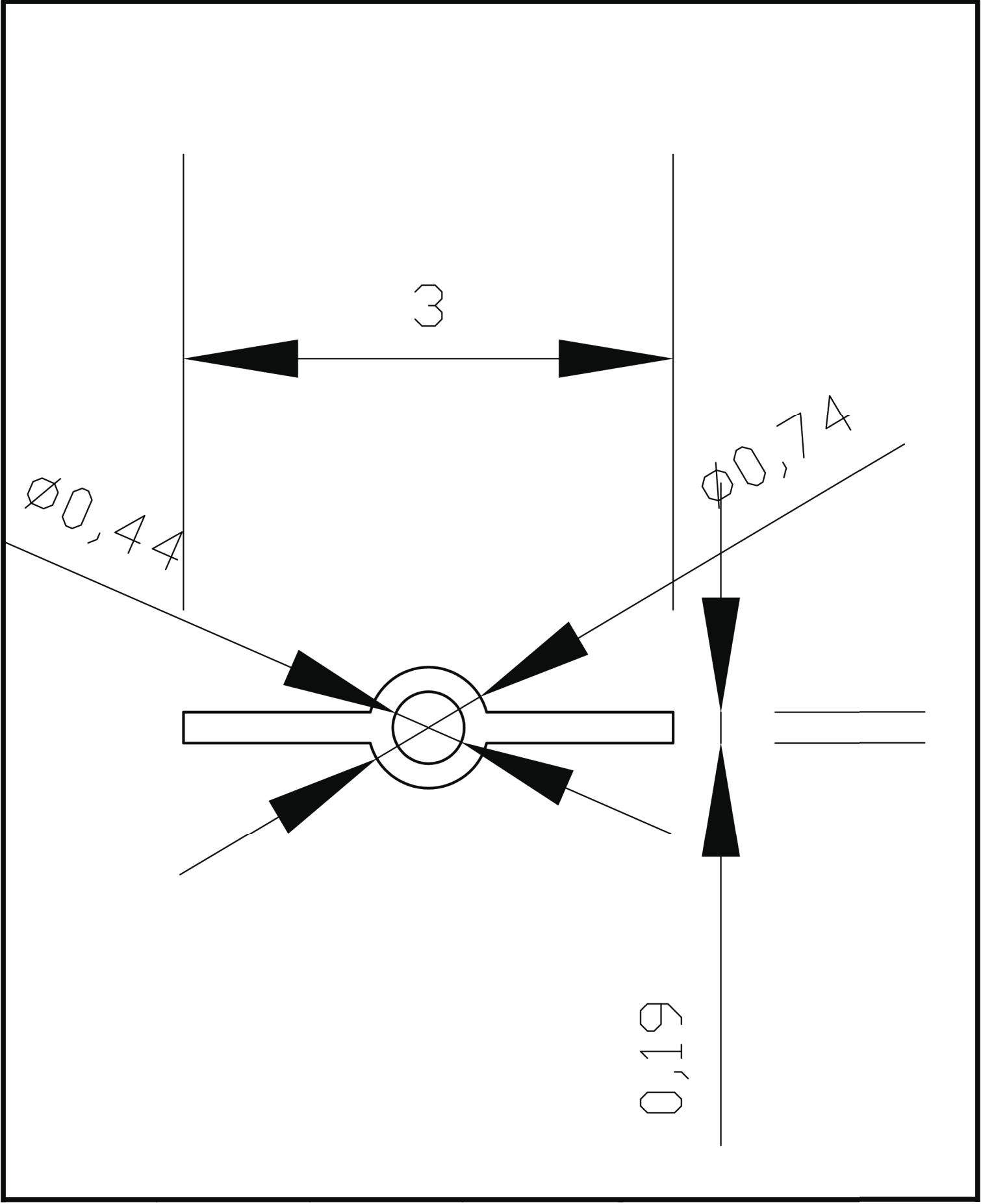
TWIST-BAND 0.44 PERFIL - PROFILE - PROFIL
